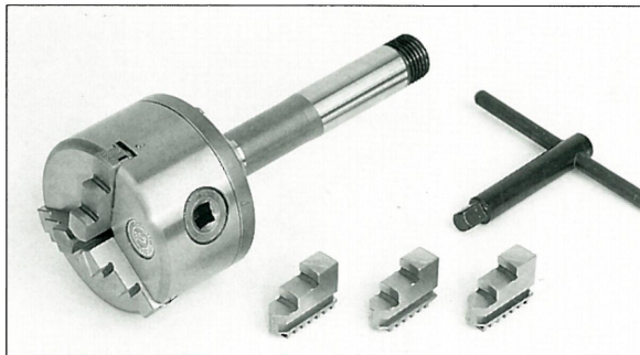
Dreibacken-Drehfutter Ø80 mm Aufspanndorn hierzu
