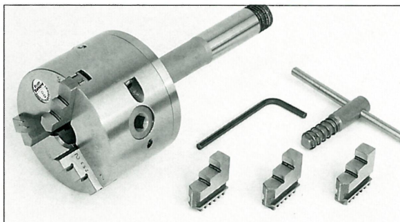
Dreibacken-Drehfutter mit 80 mm verstellbarem Zahn- kranz. Rundlauf 0,005 mm einstellbar. Aufspanndorn hierzu
