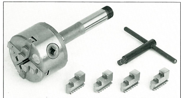
Vierbacken-Drehfutter Ø 80 mm Aufspanndorn hierzu
