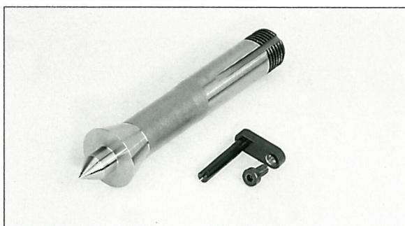
Spitze 60°
